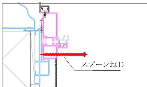
②スプーンネジ取付け断面図
